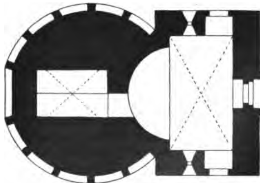
Bild 10. Grund- und Aufriß des heiligen Grabes in der Kapuzinerkirche zu Eichstätt.
